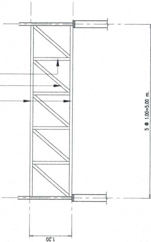
ขยาย TRUSS B มาตราส่วน 1:50
